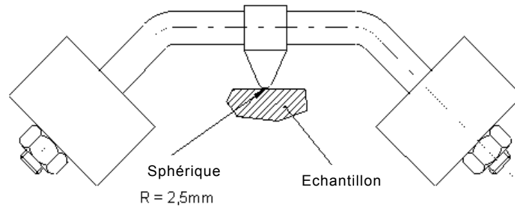
Figure 37 – Appareil pour l'essai à la bille
