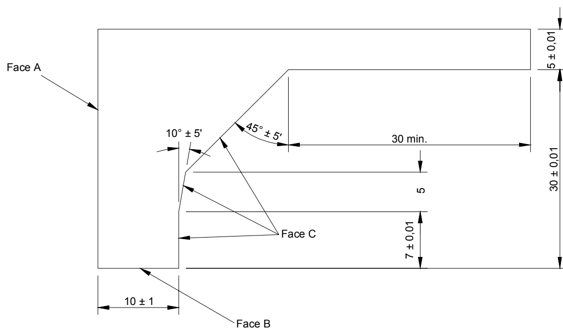
Figure 32 – Calibre (épaisseur approximative 2 mm) pour la vérification du contour des capots ou plaques de recouvrement
