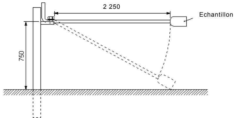
Figure 29 – Dispositif pour l'essai de la résistance mécanique des prises mobiles multiples
