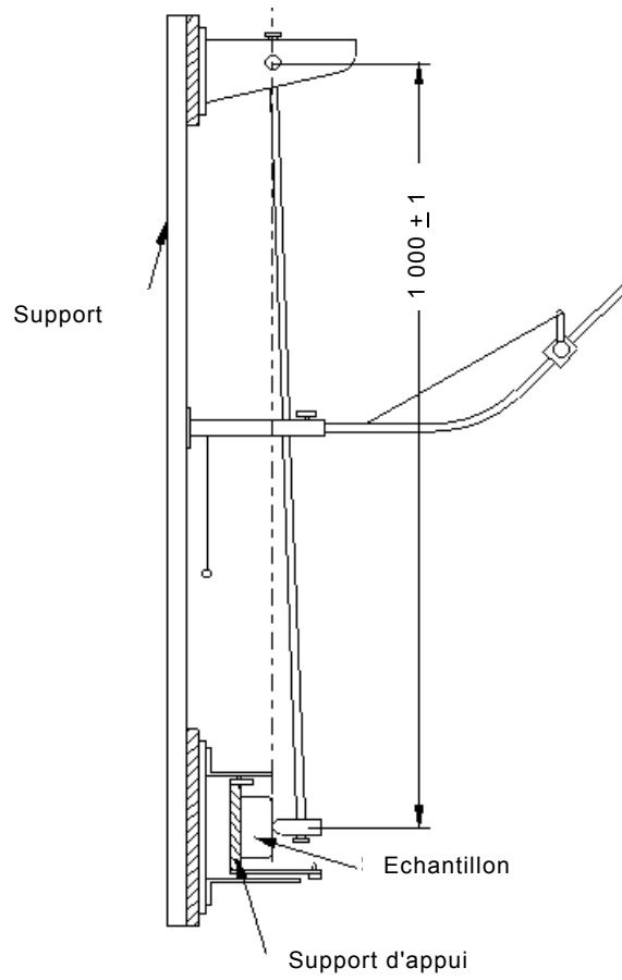
Figure 22 – Appareil d'essai de choc
