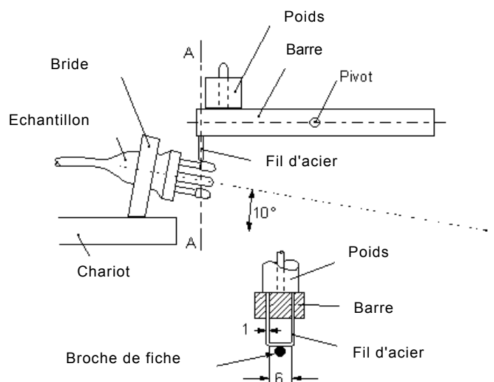
Figure 27 – Appareil d'essai de choc à basse température de 24.4
