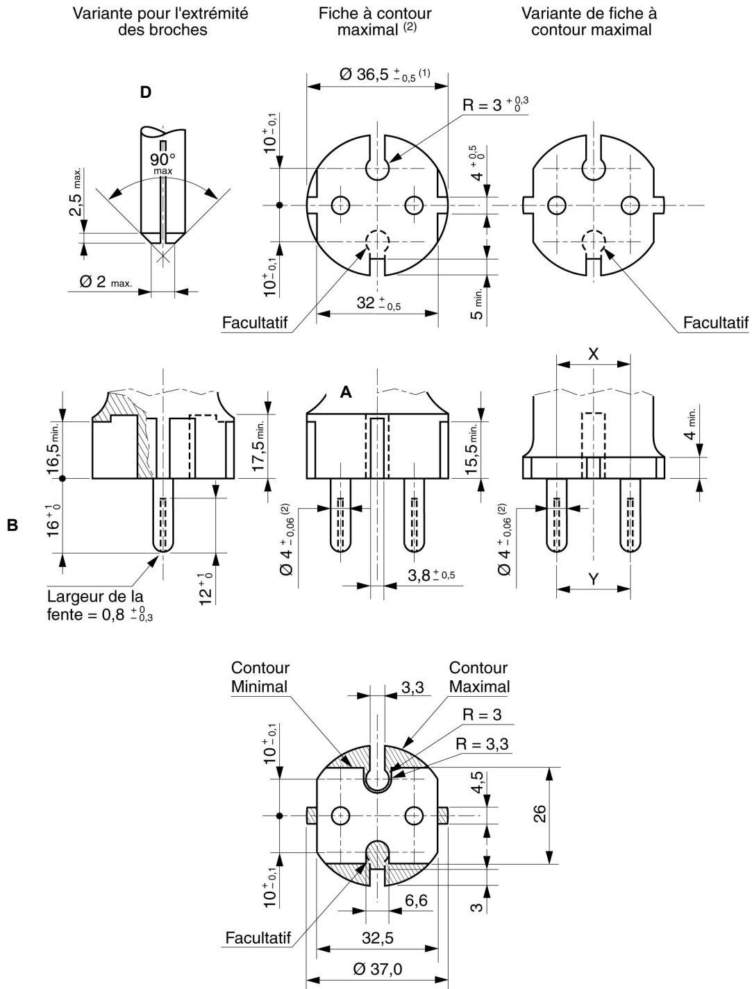
Variation admissible du contour de la surface d'engagement
