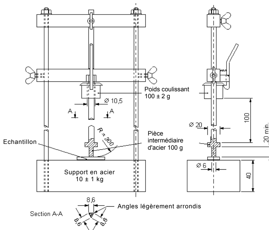
Figure 41 – Appareil pour l'essai de pression à haute température
