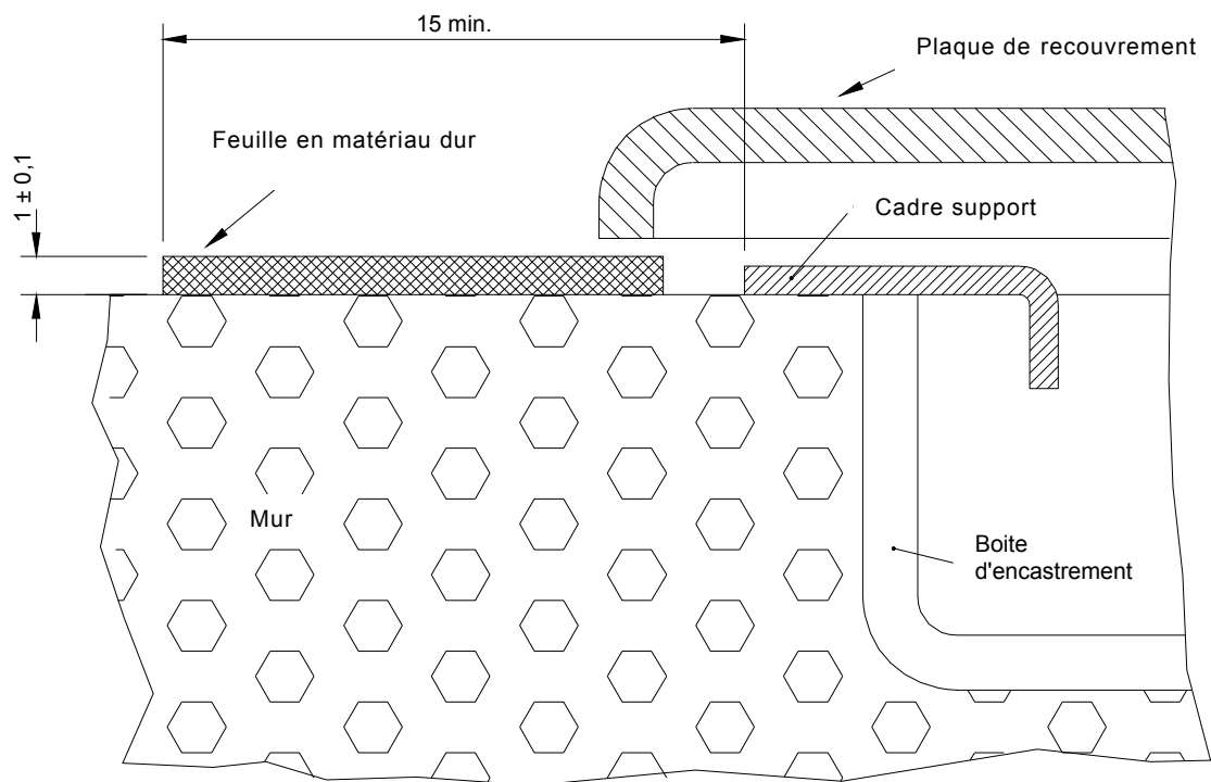
Figure 31 – Disposition pour l'essai des capots ou des plaques de recouvrement
