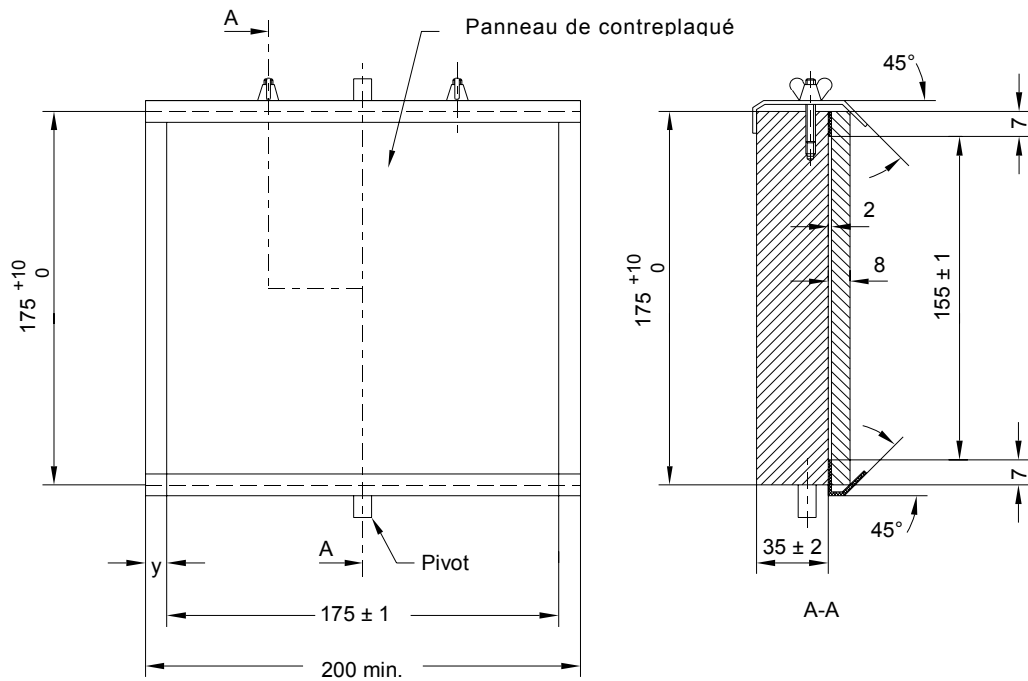
Figure 24 – Support sur lequel est fixé l'échantillon
