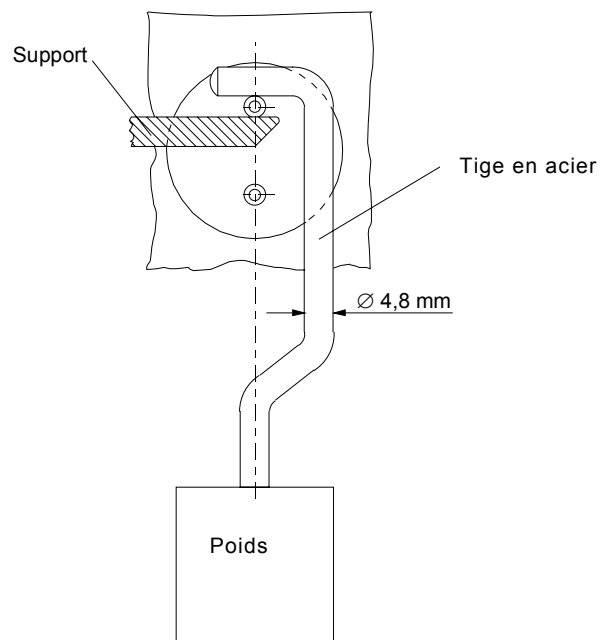
Figure 14 – Dispositif d'essai des broches non massives
