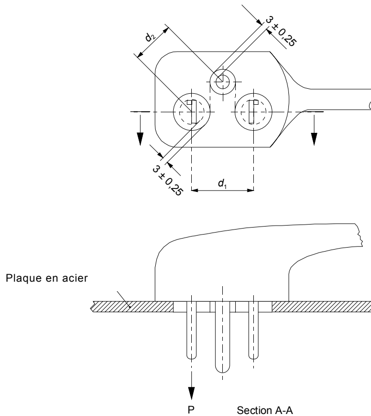
Figure 30 – Exemple de dispositif d'essai pour vérifier la fixation des broches dans le corps de la fiche
