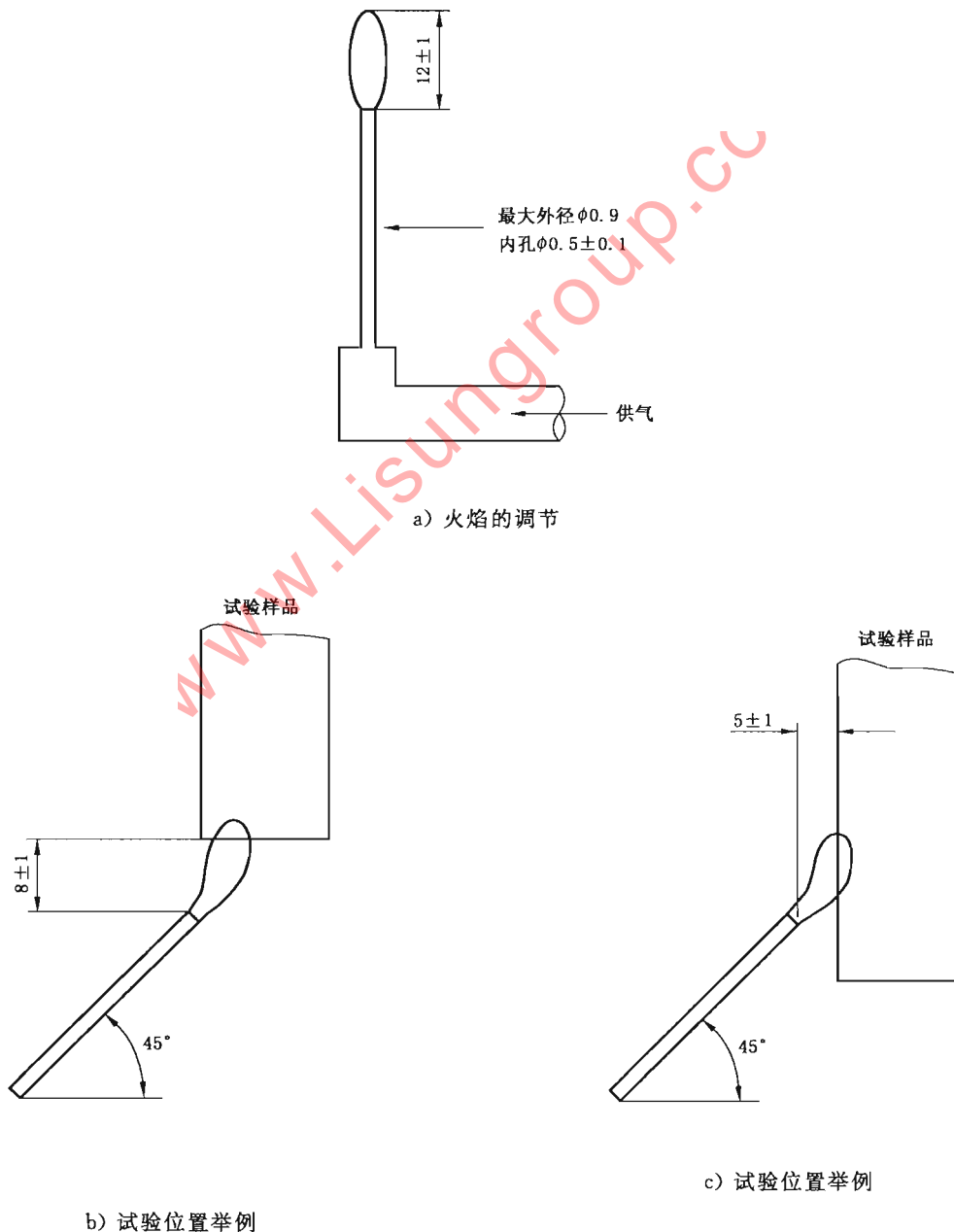
图 1 针形燃烧器
