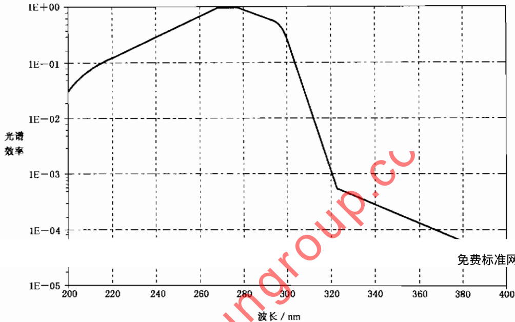
图 1 皮肤和眼睛光化学紫外危害的光谱加权函数 S_{UV}(\lambda)
