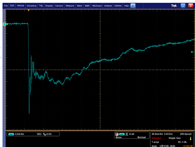
-8kV放电电流波形
